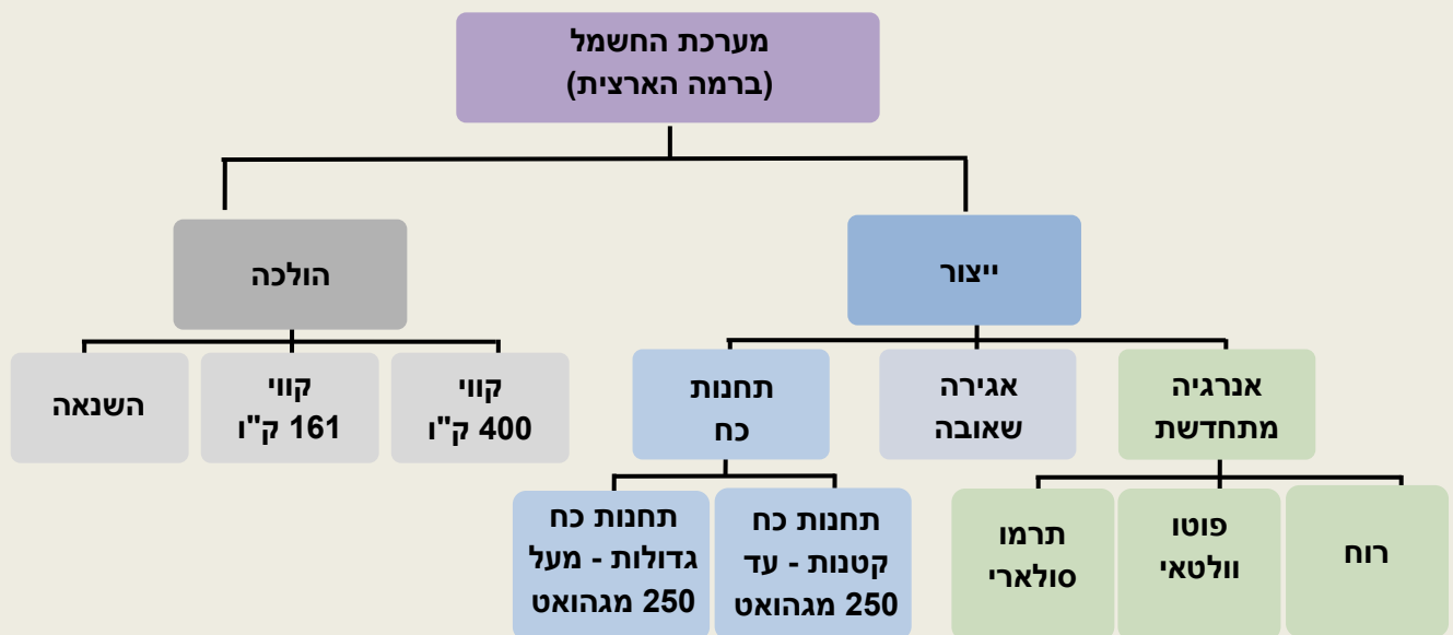
תרשים 10 - מבנה כללי של מערכת החשמל - ייצור והולכה
